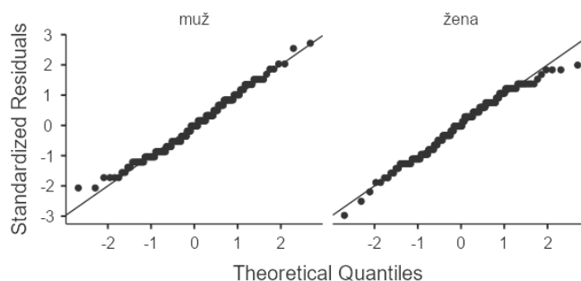
Obrázok 7.2 Q-Q grafy pre premennú Prívetivosť, samostatne pre mužov a ženy
