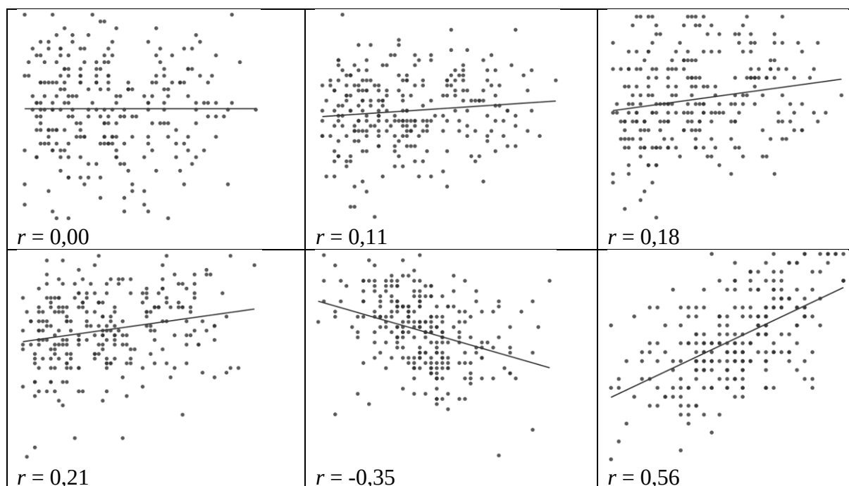
Obrázok 6.4 Grafické znázornenie vzťahov dvoch premenných (bodový graf s priamkou)
