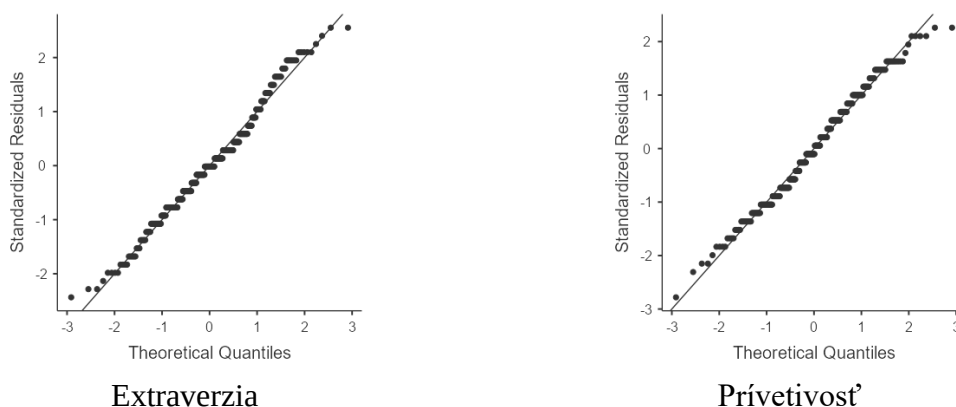
Obrázok 5.7 Q-Q grafy pre vybrané premenné
