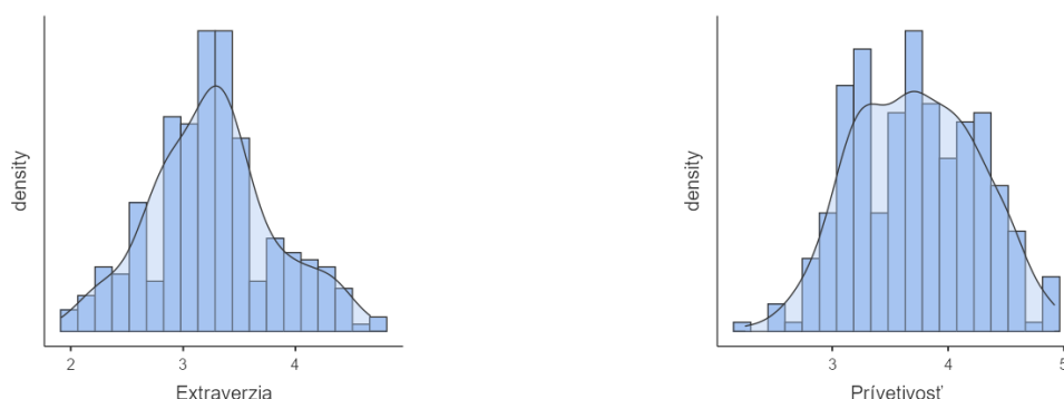
Obrázok 5.6 Histogram pre vybrané premenné
