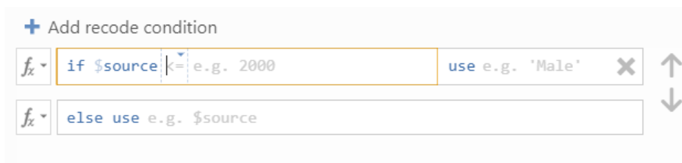
Obrázok 2.8: Panel pre nastavenie podmienenej transformácie
